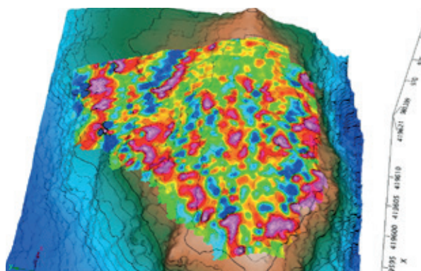
Bohinjska Česnjica – Arheološko najdišče Dunaj pri Trebež. Rezultati magnetnih meritev na 3D prikazu lidarske topografije (izdelal: I. Medarić).
