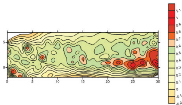
Kaštelir pri Čedljah (EŠD 7238). Rezultati kartiranja navidezne magnetne susceptibilnosti.
