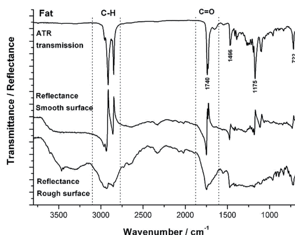
Slika 5. FTIR spekter maščobe (Prinsloo et al. 2014, 736, sl. 6c).
