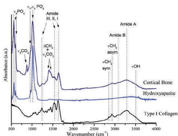
Slika 4. FTIR spektri kortikalne kosti, hidroksiapatita in kolagena tipa I (Figueiredo et al. 2014, 321, sl. 4).
