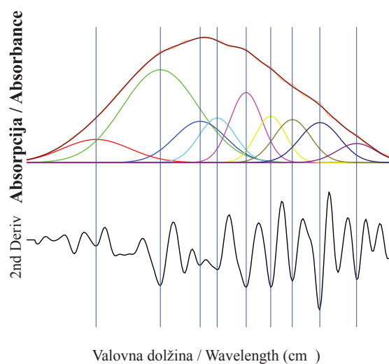
Slika 11. Odvajanje in pridobitev posameznih komponent traku amida I.
