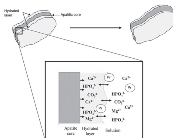
Slika 3. Hidrirani sloj na površini kristala (Farlay et al. 2010, 334, sl. 1).
