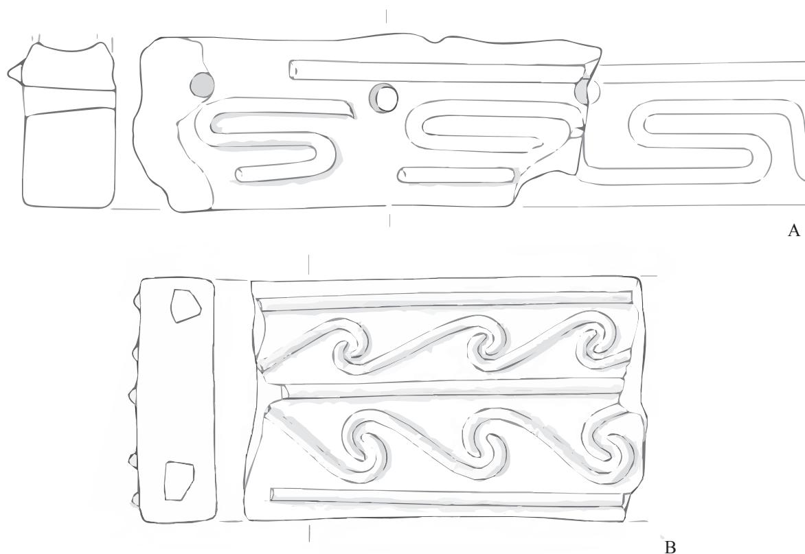
Slika 9. Stenska glinena obloga z navpičnim (A) in vodoravnim (B) načinom pritrdjevanja (po Svoljšak, Dular 2016, T. 5: 1; 87: 1).
